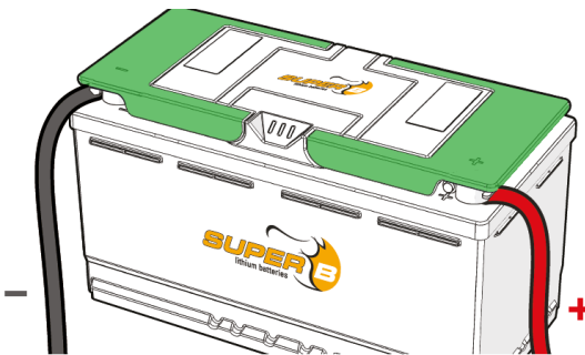
Figuur 8. Plaats de handgrepen over de aansluitklemmen
