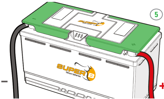
Figuur 11. Plaats de handgrepen over de aansluitklemmen
